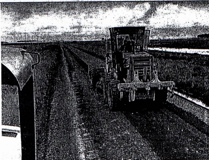
- UR 203 E 205 - BRETE PASSO DO VAI, DA ESTÂNCIA DOM PATRÍCIO PASSANDO PELA ESTÂNCIA CORUNILHA EM DIREÇÃO A SANGA DO VAI
