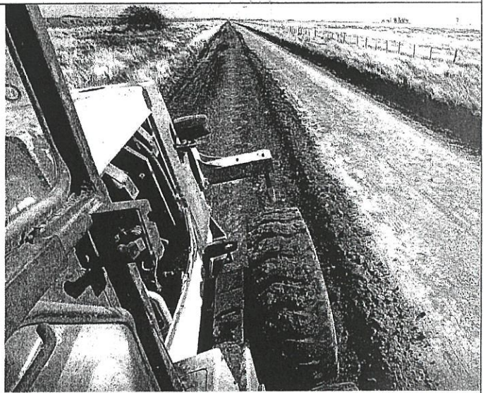
- UR 418 - BRETE DO ADOLF STERN DA VILA DO PLANO ALTO EM DIREÇÃO AO PASSO DO CEMITÉRIO
