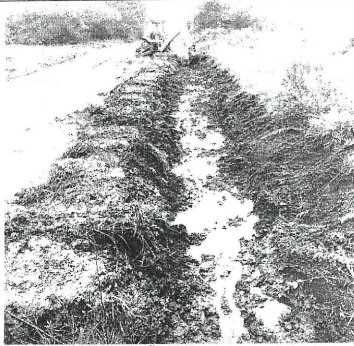
UR 201 - VILA DE JOÃO ARRREGUI, FOI REALIZADO TRAVESSIA DE BUEIROS, LIMPEZA DE VALAS E COLOCAÇÃO DE MATERIAL EM 13 QUILOMETROS
