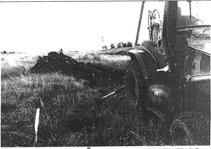
JR 201 - VILA DE JOÃO ARRREGUI, FOI REALIZADO TRAVESSIA DE BUEIROS, LIMPEZA DE VALAS E COLOCAÇÃO DE MATERIAL EM 13 QUILOMETROS
