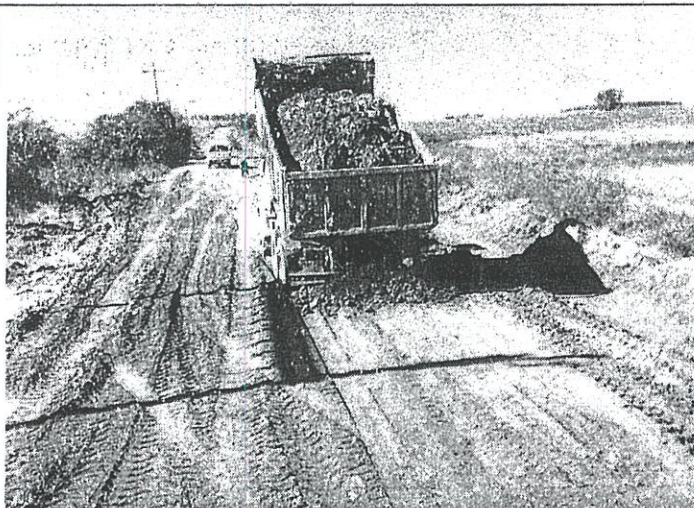
UR 101 - BRETE DO CHAPADAO, DA ESTÂNCIA MEIA ÁGUA EM DIREÇÃO A CAPELA DO IPANÉ
