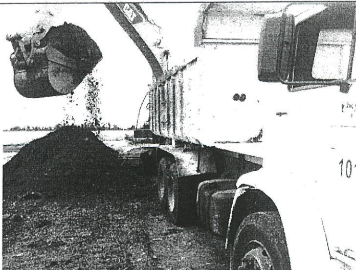
JR 201 - VILA DE JOÃO ARRREGUI, FOI REALIZADO TRAVESSIA DE BUEIROS, LIMPEZA DE VALAS E COLOCAÇÃO DE MATERIAL EM 13 QUILOMETROS
