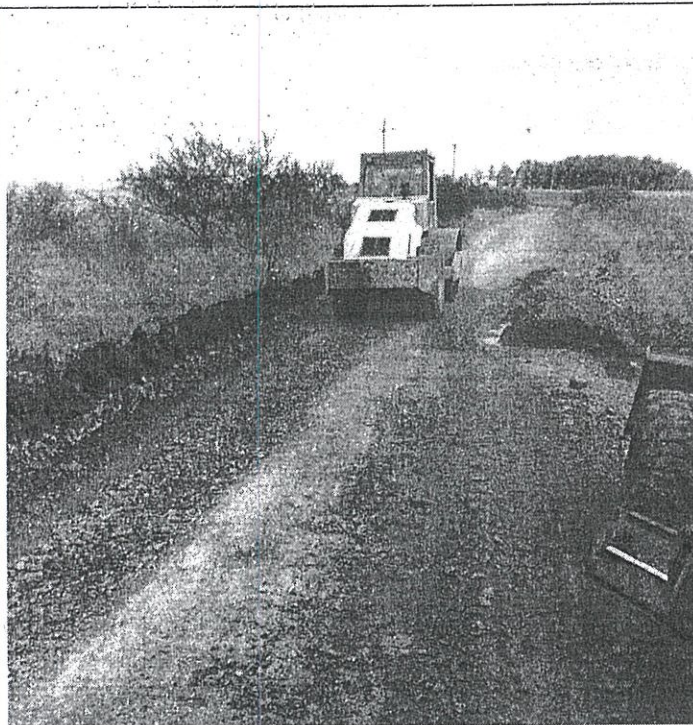
UR 101 - BRETE DO CHAPADAO, DA ESTÂNCIA MEIA ÁGUA EM DIREÇÃO A CAPELA DO IPANÉ
