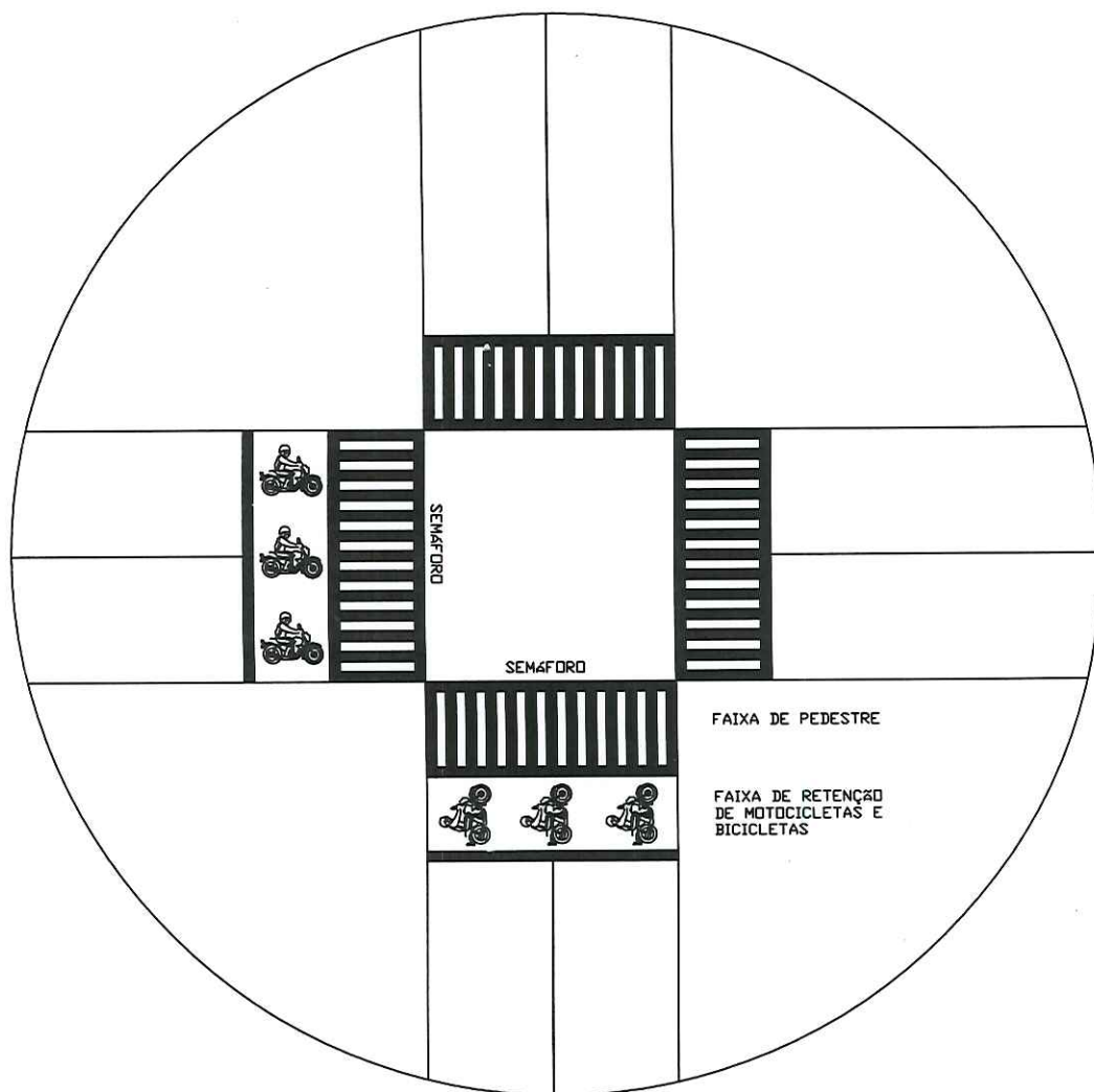
DETALHE CRUZAMENTO COM SEMÁFOROS E INSTALAÇÃO DE FAIXA DE RETENÇÃO PARA MOTOCICLETAS E BICICLETAS
